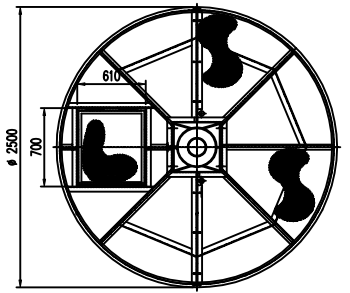
PIATTAFORMA FISSA (TIPICA) FIXED PLATFORM (TYPICAL)
