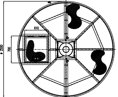
SEZIONE 'C-C' SECTION 'C-C'
