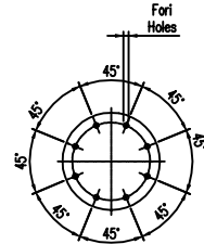
CONTROFLANGIA MASK PLATE
