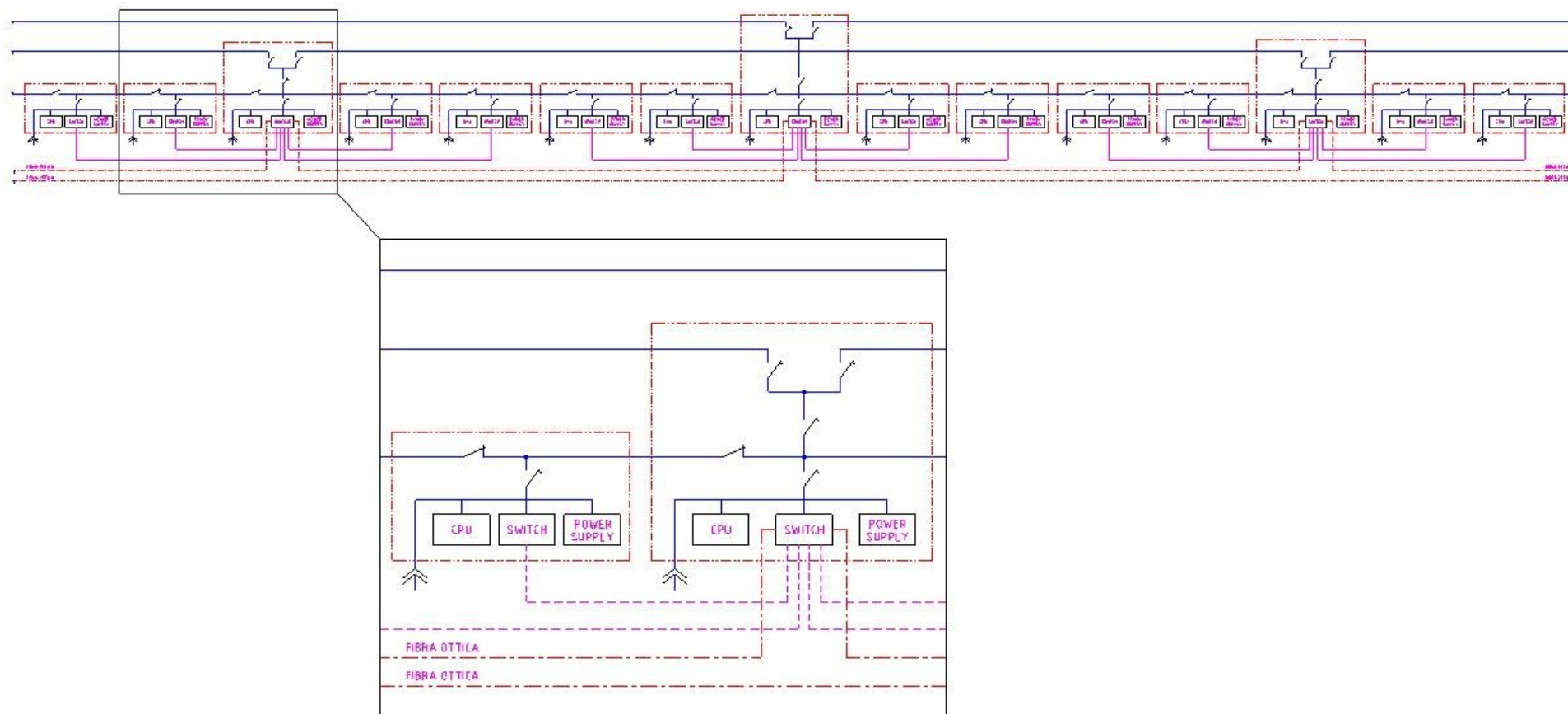
Schema tipico dei collegamenti elettrici e di segnale con doppio anello ridondante
