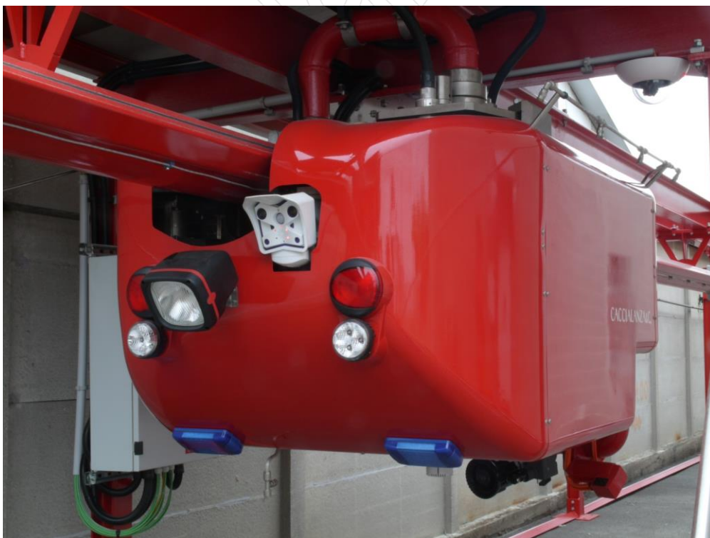
Fotografia della unità mobile (carrello monitoratore) collegata alla stazione
