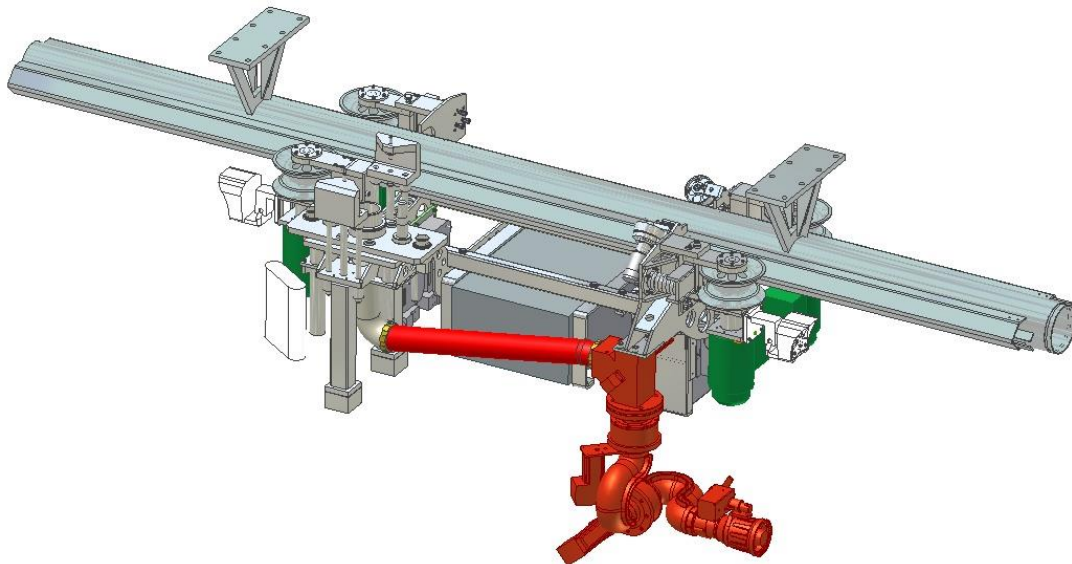
Schema unità mobile (carrello monitoratore) con cofano rimosso
